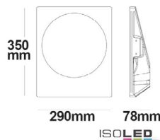
112166 | Gips-Wand-Einbauleuchte, GU10, große Öffnung rund
