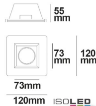
112075 | Gips-Einbaustrahler GU5.3, quadratisch mit Glas satin,
