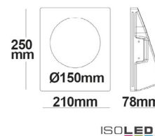
112177 | Gips-Decken-Anbauleuchte, GU10, rund
