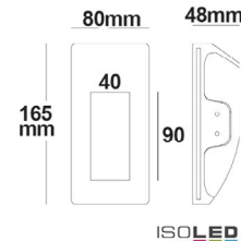
112168 | Gips-Wand-Einbauleuchte, länglich, GU10, große
